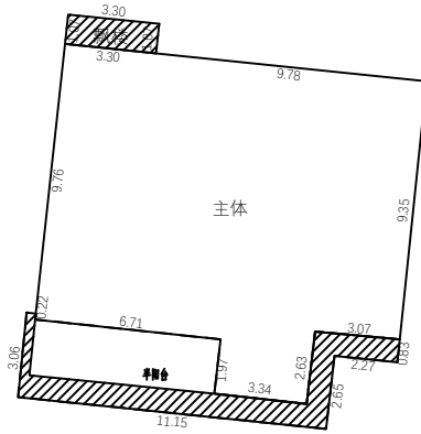
2层平面图
