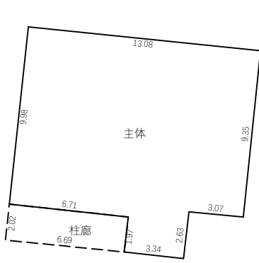
1层平面图
