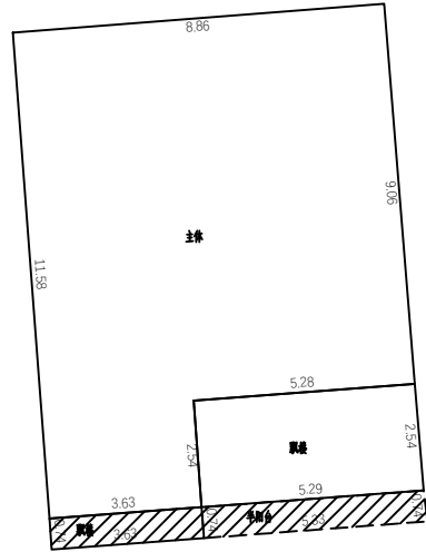
2层平面图
