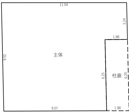
1层平面图
