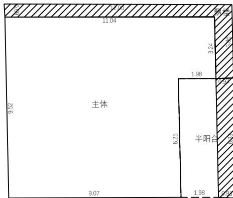
3层平面图
