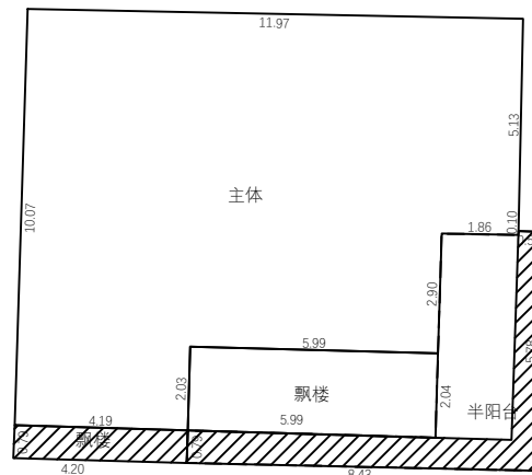
2层平面图
