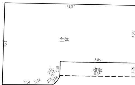
3层平面图
