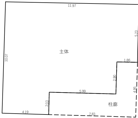
1层平面图
