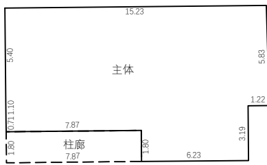
1层平面图
