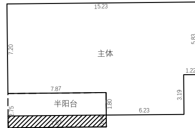
2层平面图
