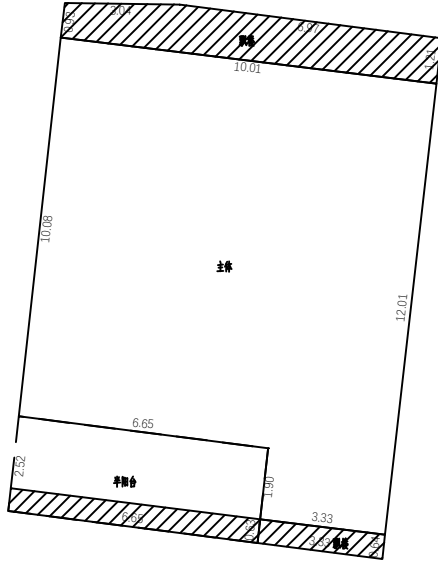
3层平面图
