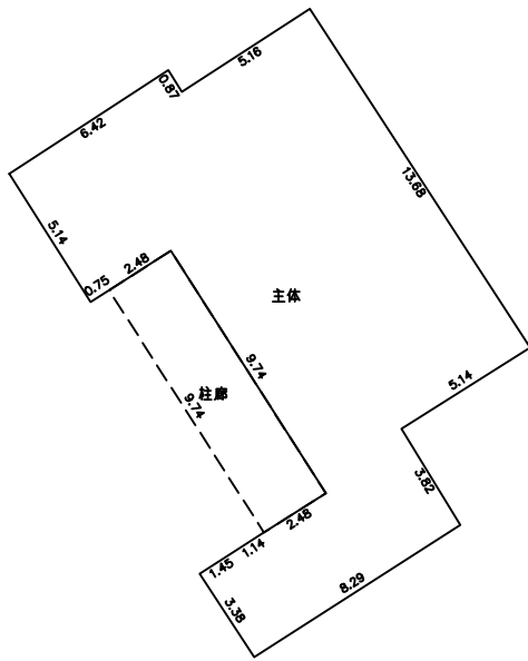
第1层平面图
