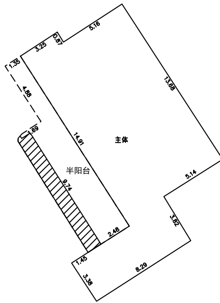
第2层平面图
