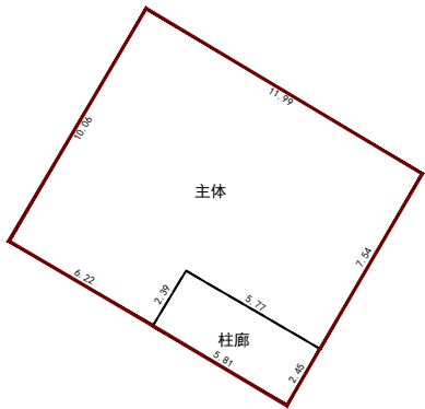
第1层平面图
