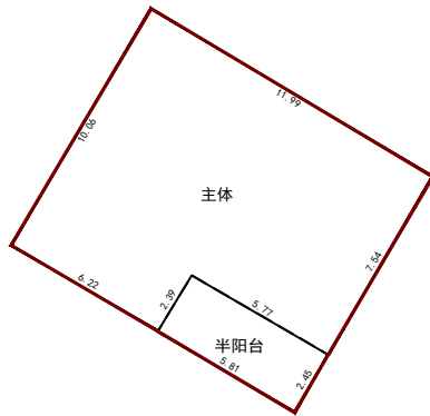
第2层平面图
