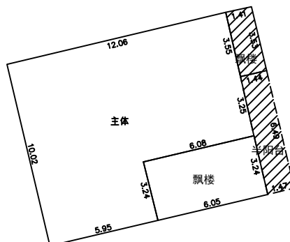
第2?平面?
