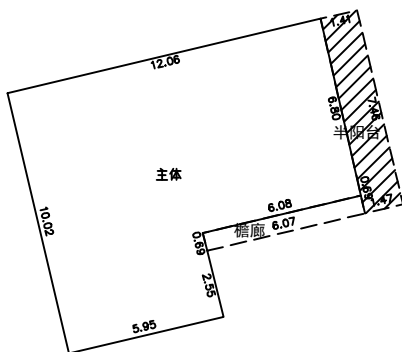
第3层平面图
